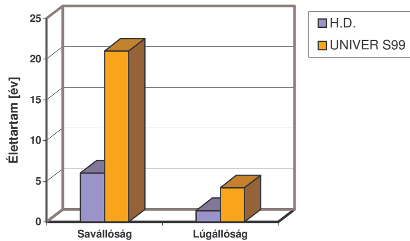
3.ábra: Kémiai ellenállókéesség szerinti élettartam változás
